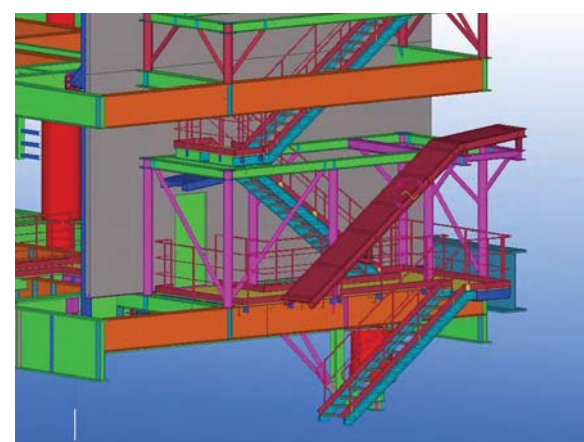
塔楼雨棚斜梯
