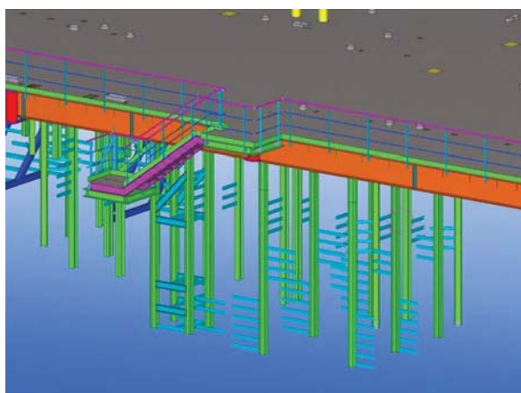
电仪支架
