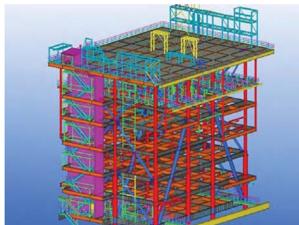
模块模型
