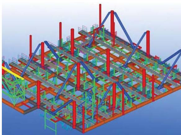
整层模型
