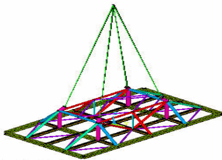
吊装框架设计
