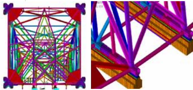
番禺30-1导管架立片ANSYS模型
