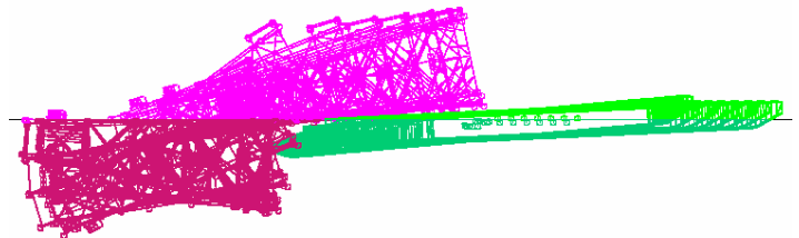
乐东导管架下水分析
