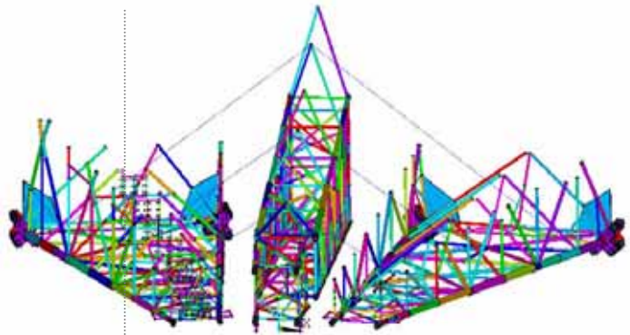
番禺30-1导管架立片方案之一
